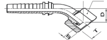
TE0120 PAG. METRIC DIN LIGHT FEMALE SWIVEL (24° CONE SEAT) - 45° ELBOW
